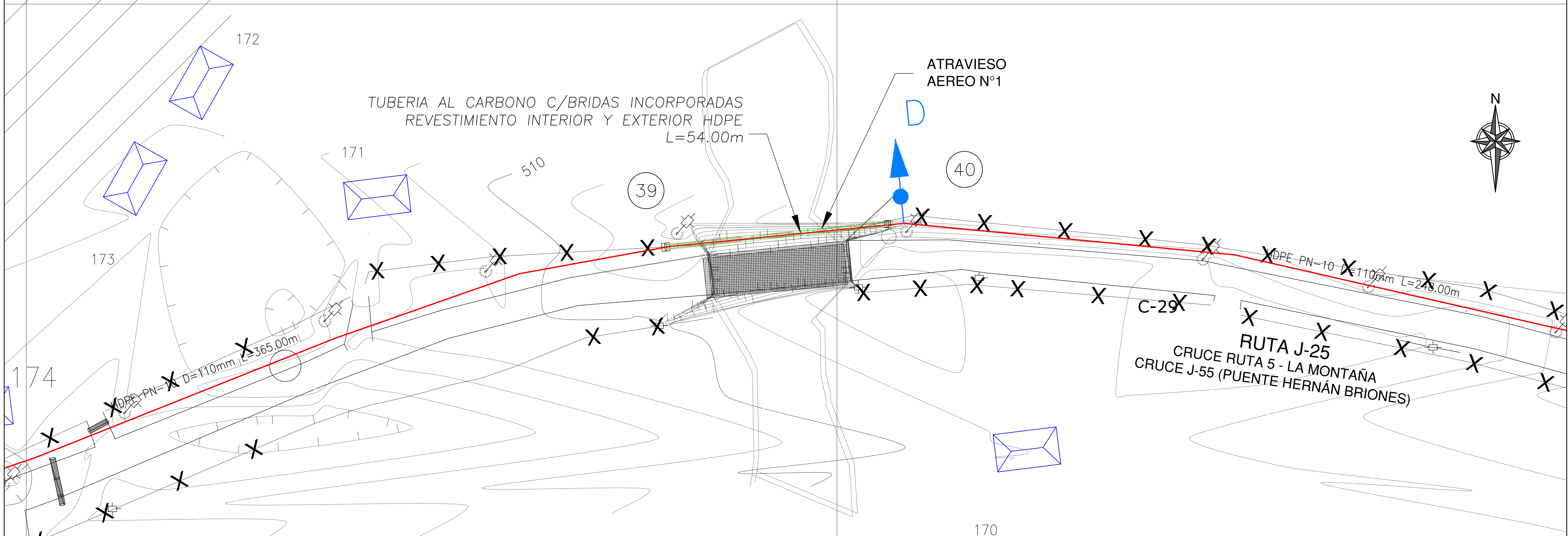
PLANTA ATRAVIESO N°1 ESCALA 1 : 500
