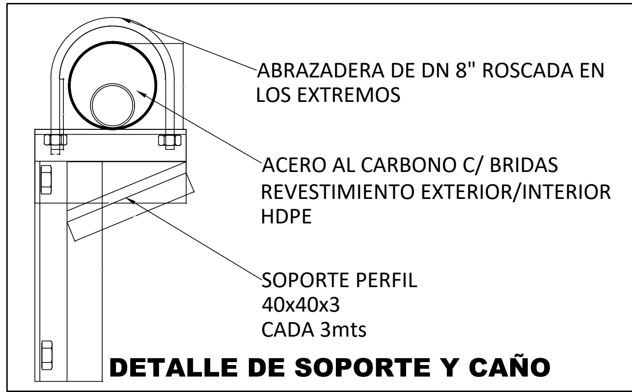
DETALLE DE SOPORTE Y CAÑO
